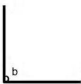
Right angle : b = 90^\circ
