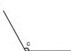
Obtuse angle : 90^\circ < c < 180^\circ
