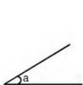
Acute angle : 0^\circ < a < 90^\circ
